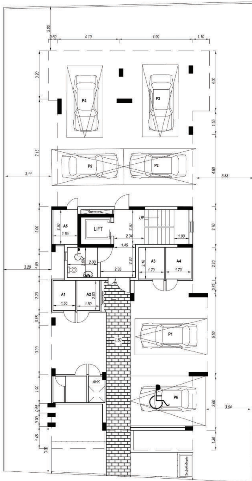
ΚΑΤΟΨΗ ΥΠΟΣΤΕΓΟΥ GROUND FLOOR PARKING
